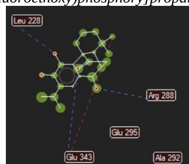
Rosmanol
