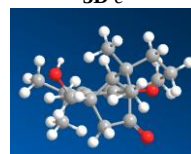
Rosmanol 3D
