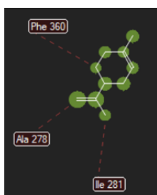
Limonene
